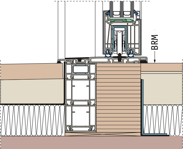
Hebeschiebetür-Flügel
