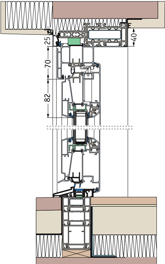
Haustür mit Schwelle
