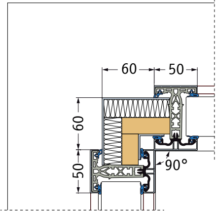
schmale Inneneckkoppelung 90°
