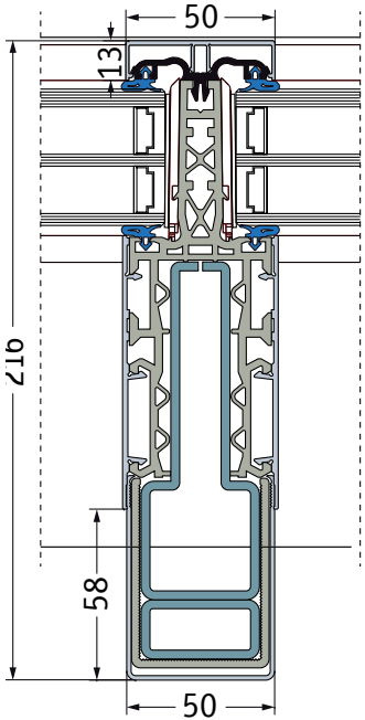
Code P4 max. Höhe ca. 4.000 mm
