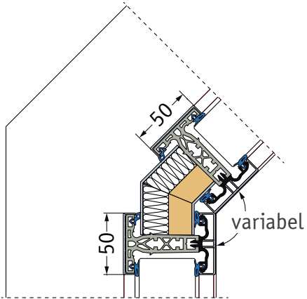
schmale Inneneckkoppelung variabel
