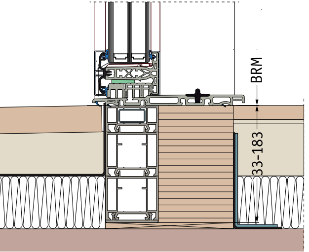
Festverglasung mit Führungs- schienen Hebeschiebetür-Flügel
