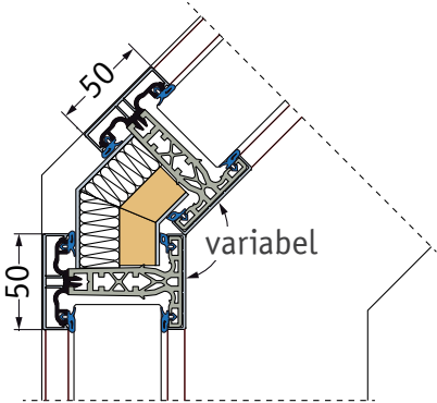
schmale Eckkoppelung variabel
