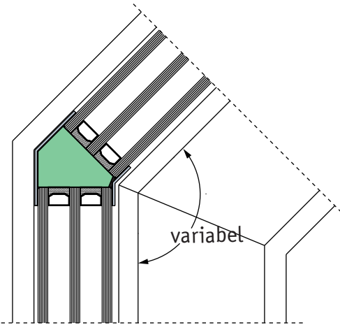
Glasecke variabel
