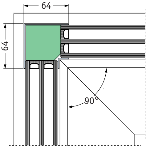
Glasecke 90°
