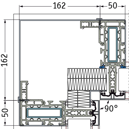
Inneneckkoppelung 90°
