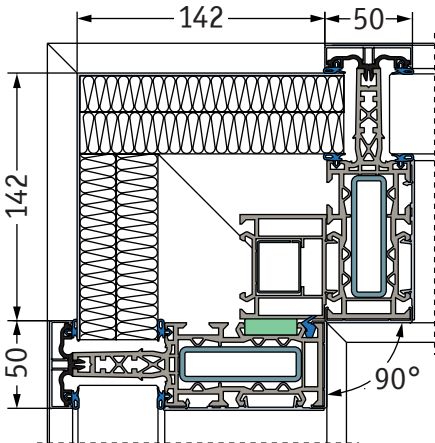
Eckkoppelung 90°
