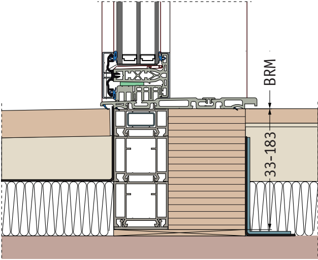
Festverglasung
