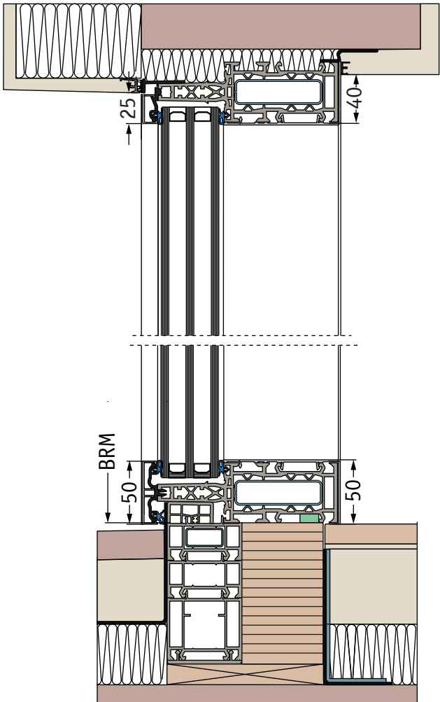
Seitenteil mit Blendrahmen unten
