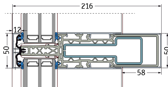
Code R3 max. Höhe ca. 3.800 mm
