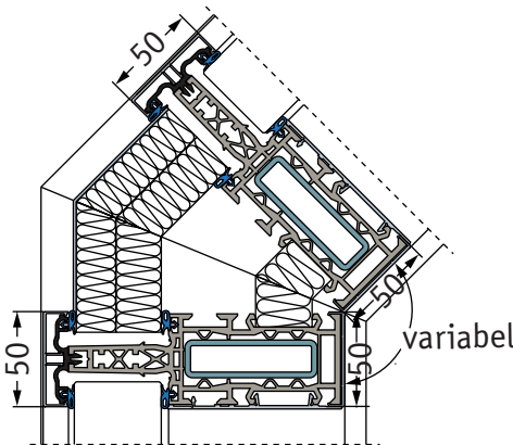
Eckkoppelung variabel
