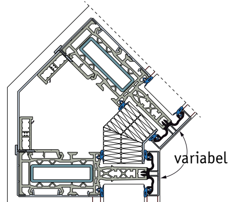
Inneneckkoppelung variabel
