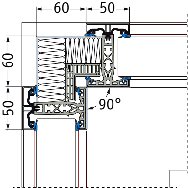
schmale Eckkoppelung 90°
