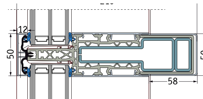
Code R4 max. Höhe ca. 4.000 mm
