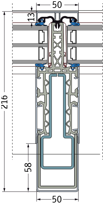
Code P3 max. Höhe ca. 3.800 mm
